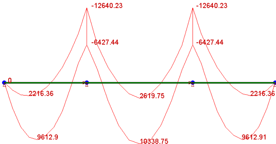
Enveloppe pondérée de la flexion (Combinaison de charges #1)
