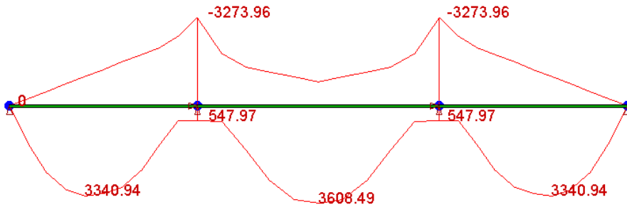
Enveloppe de la flexion pour la charge mobile de voie
